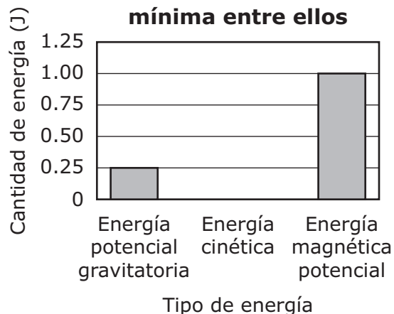
B. Energía cuando los carros estaban a la distancia mínima entre ellos
